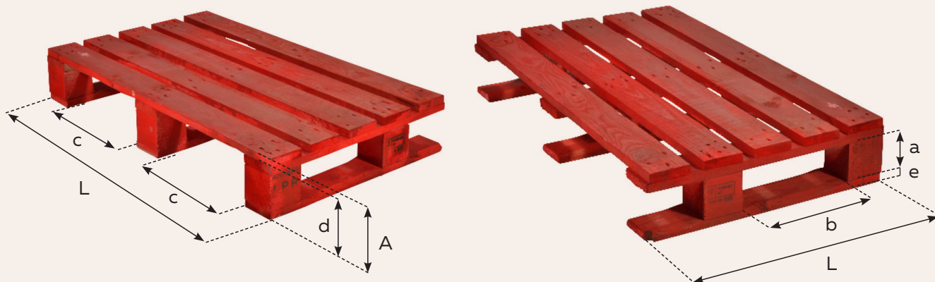
DP610 - Dimensioni nominali del pallet e tolleranza (mm)
