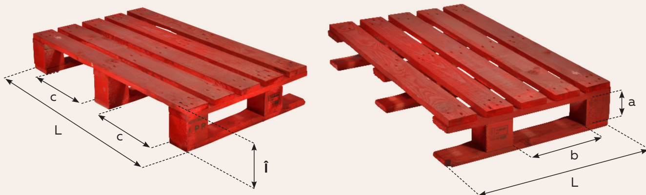
DP610 - Dimensiuni nominale și toleranța paletilor (mm)
